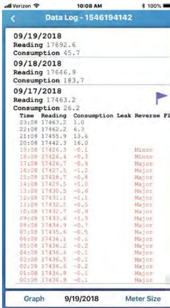
Figure 25 - Relevés heure par heure du journal de données
